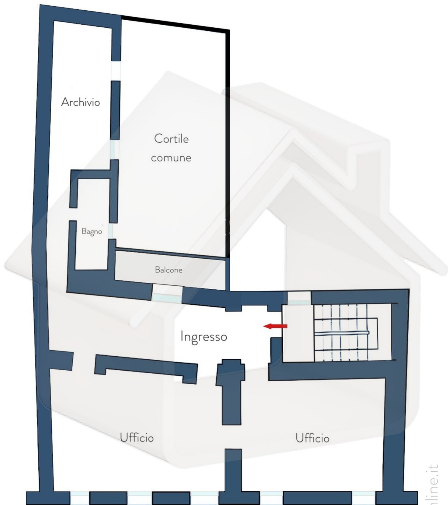
PIANTA PIANO SECONDO h: 2.70
