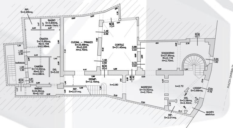
PIANO PRIMO
