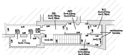
PIANO PRIMO
